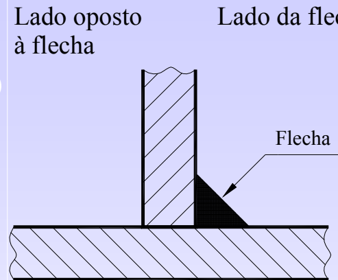
a) Soldadura do lado da flecha
